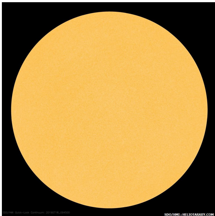
Слънчевият диск на 18 юли 2019г (SDO/HMI)
