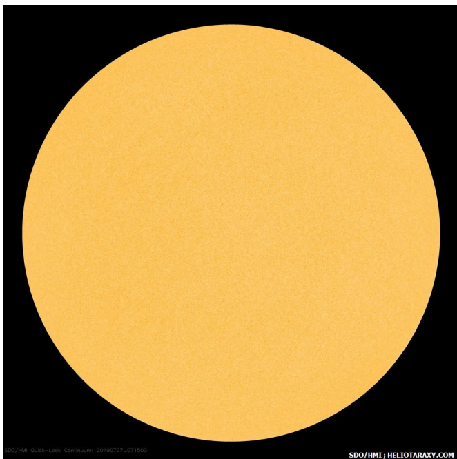
Слънчевият диск на 27 юли 2019г (SDO/HMI)
