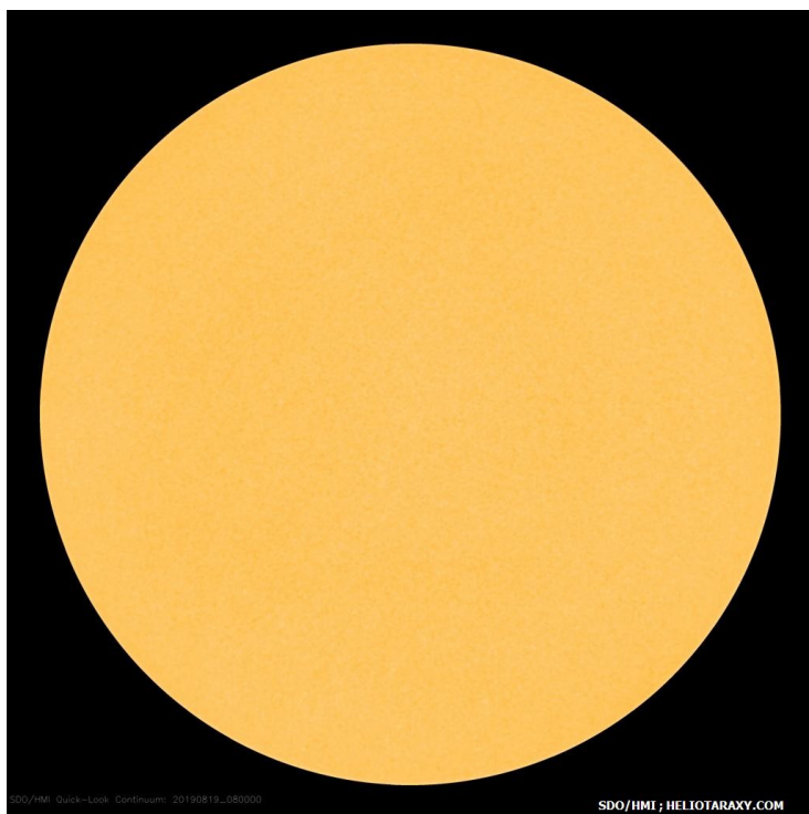
Слънчевият диск на 19 август 2019г (SDO/HMI)
