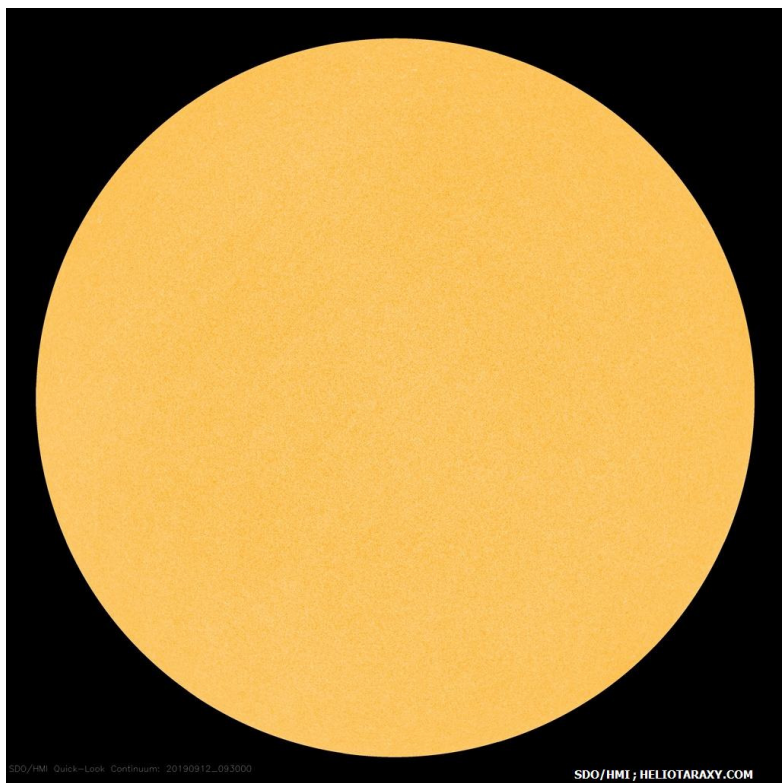
Слънчевият диск на 12 септември 2019г (SDO/HMI)
