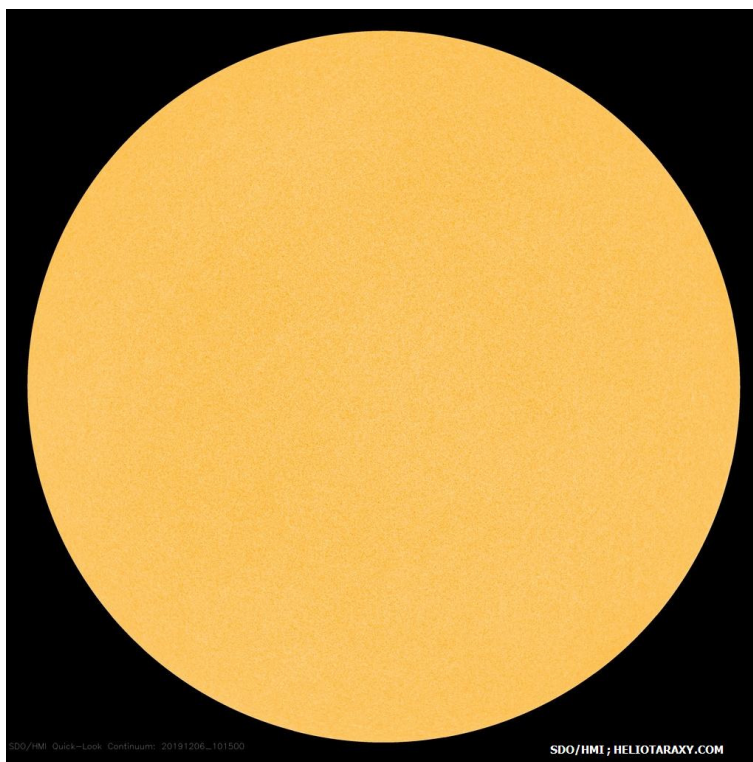
Слънчевият диск на 06 декември 2019г (SDO/HMI)
