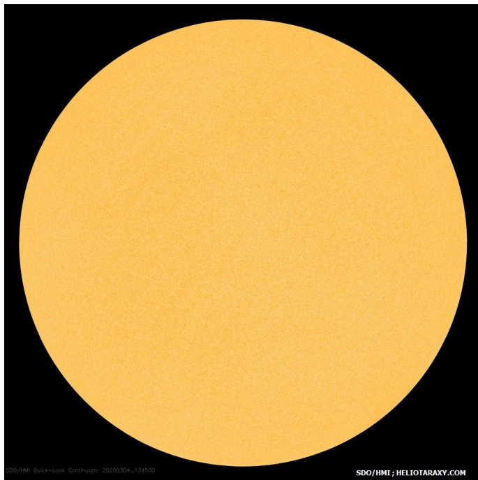
Слънчевият диск на 04 март 2020г (SDO/HMI)
