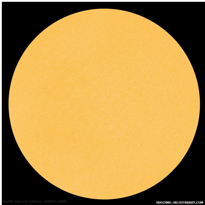
Слънчевият диск на 16 март 2020г (SDO/HMI)
