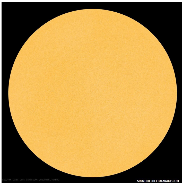
Слънчевият диск на 16 април 2020г (SDO/HMI)
