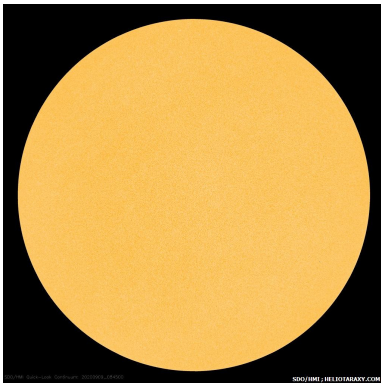
Слънчевият диск на 09 септември 2020г (SDO/HMI)
