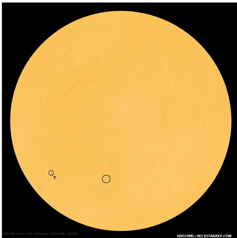
Слънчевият диск на 08 октомври 2020г (SDO/HMI)
