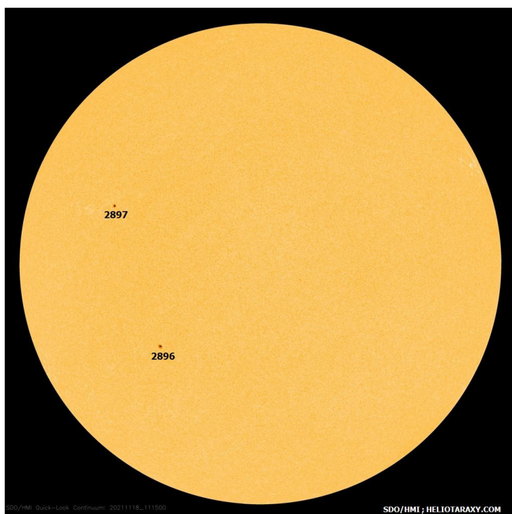
Слънчевият диск на 18 ноември 2021г (SDO/HMI)
