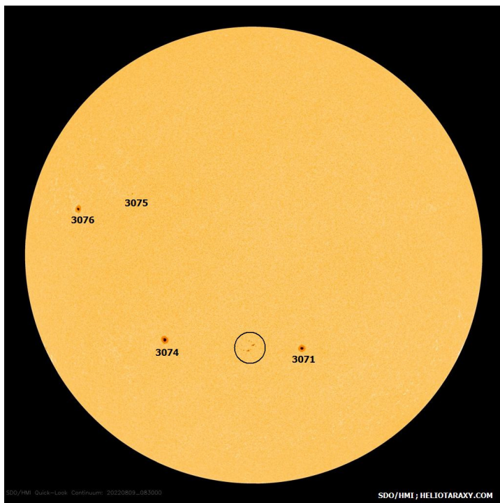
Слънчевият диск на 09 август 2022г (SDO/HMI)
