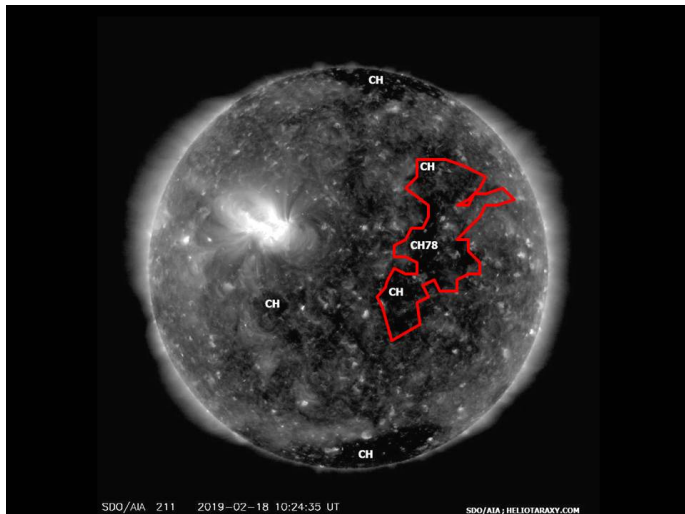
Слънчевите коронални дупки на 18 февруари 2019г (SDO/AIA)
