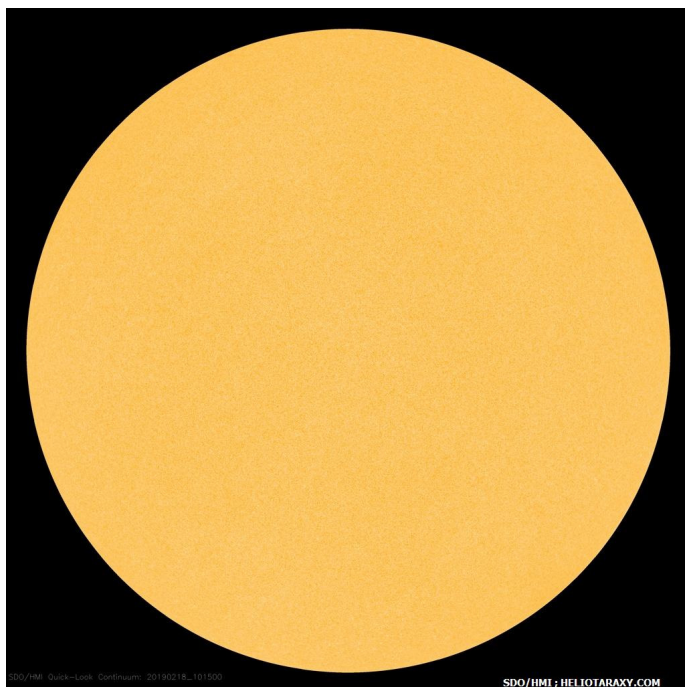
Слънчевият диск на 18 февруари 2019г (SDO)
