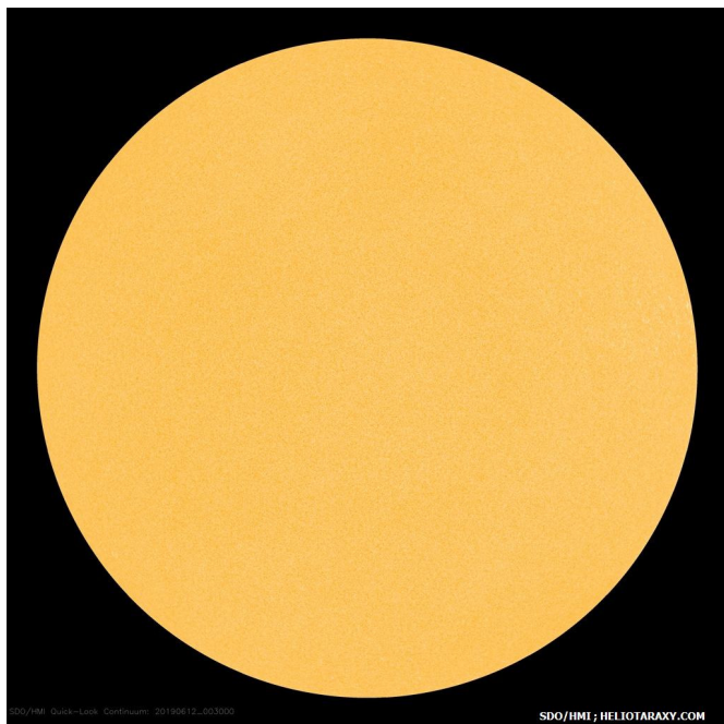
Слънчевият диск на 17 юни 2019г (SDO/HMI)
