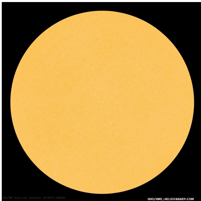
Слънчевият диск на 21 юли 2019г (SDO/HMI)
