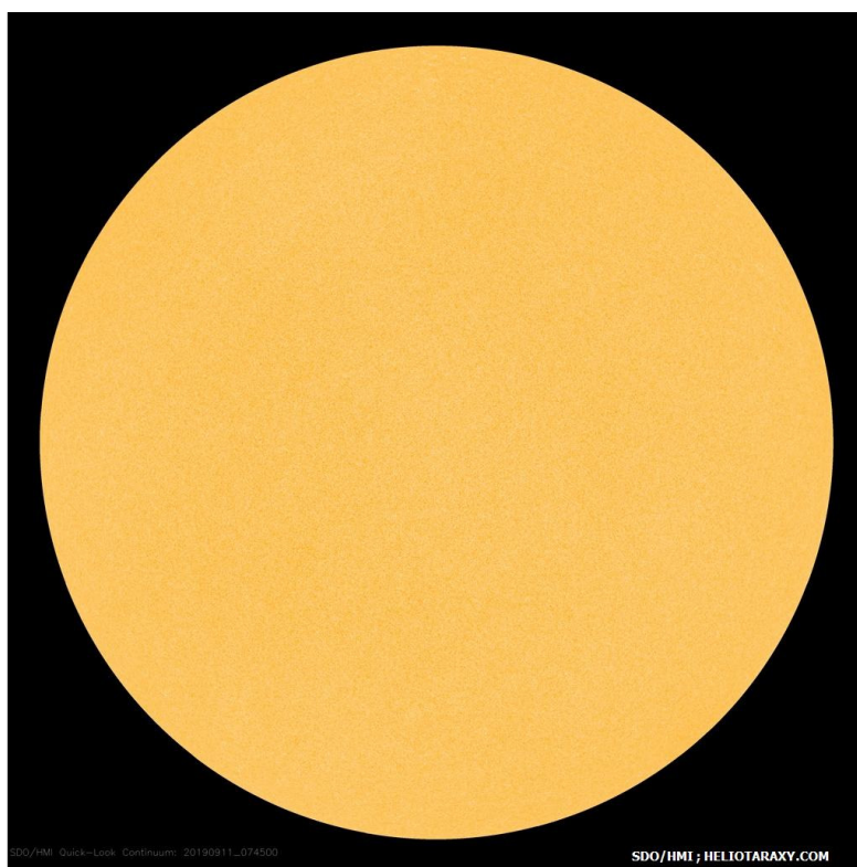
Слънчевият диск на 11 септември 2019г (SDO/HMI)
