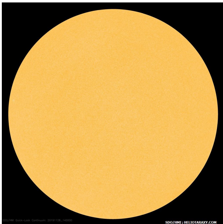
Слънчевият диск на 28 ноември 2019г (SDO/HMI)
