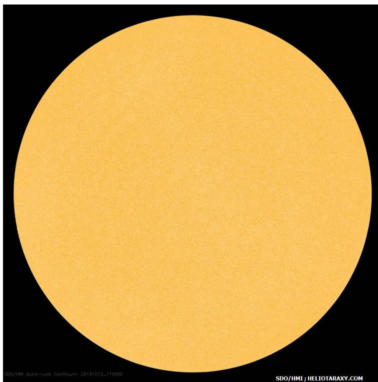
Слънчевият диск на 13 декември 2019г (SDO/HMI)
