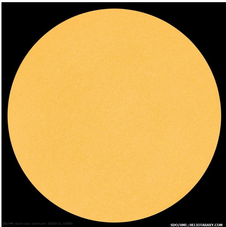
Слънчевият диск на 23 януари 2020г (SDO/HMI)
