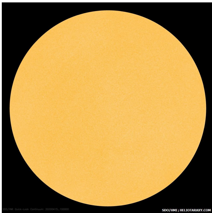
Слънчевият диск на 15 април 2020г (SDO/HMI)
