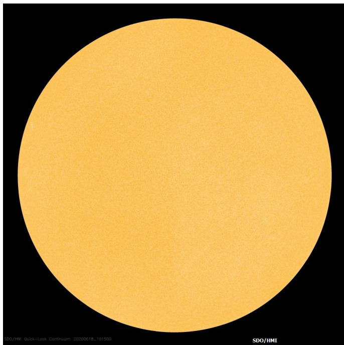
Слънчевият диск на 18 юни 2020г (SDO/HMI)
