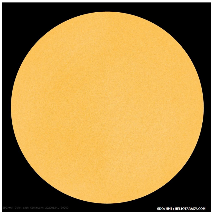
Слънчевият диск на 24 юни 2020г (SDO/HMI)
