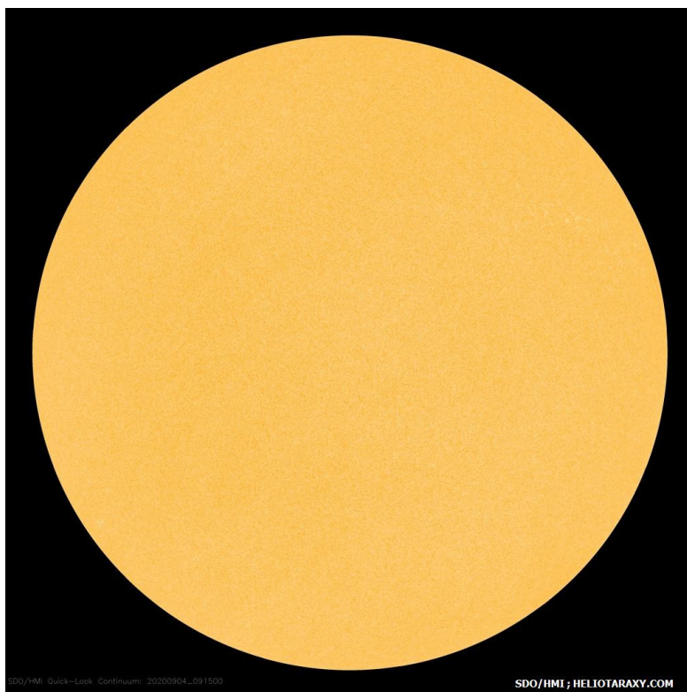
Слънчевият диск на 04 септември 2020г (SDO/HMI)
