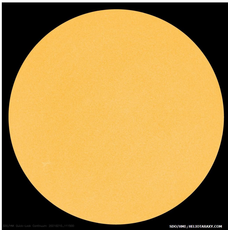
Слънчевият диск на 10 февруари 2021г (SDO/HMI)
