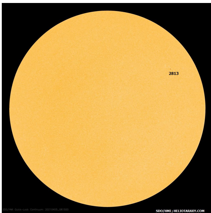
Слънчевият диск на 05 април 2021г (SDO/HMI)
