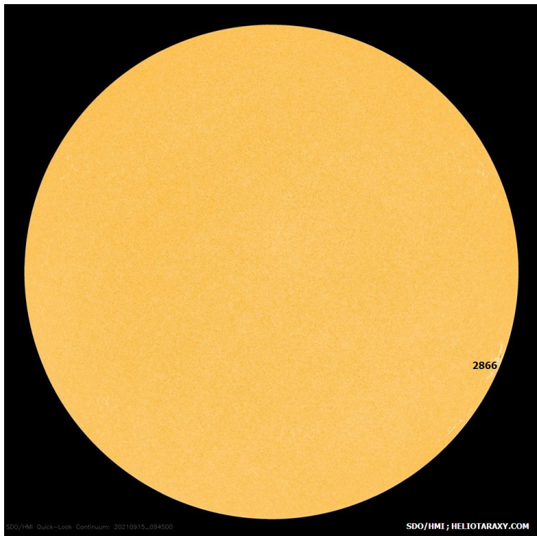
Слънчевият диск на 15 септември 2021г (SDO/HMI)
