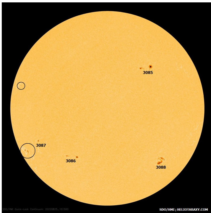
Слънчевият диск на 25 август 2022г (SDO/HMI)
