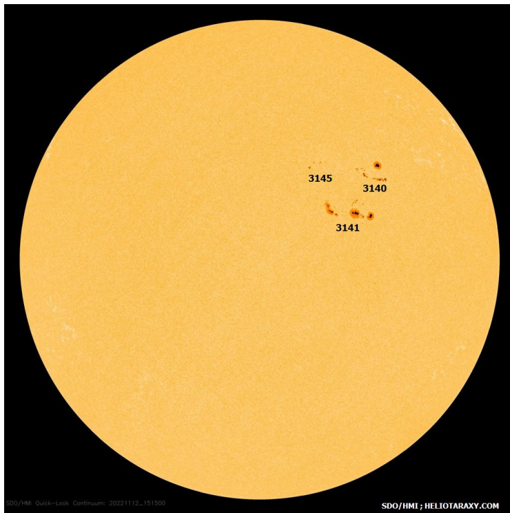
Слънчевият диск на 12 ноември 2022г (SDO/HMI)
