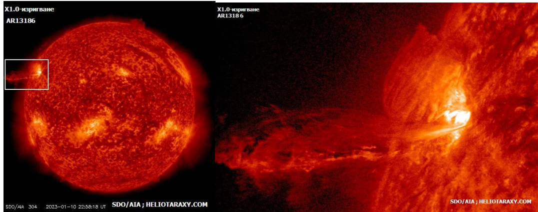
Слънчево X1.0-изригване в активната област AR13187 (3187) (SDO/AIA)
