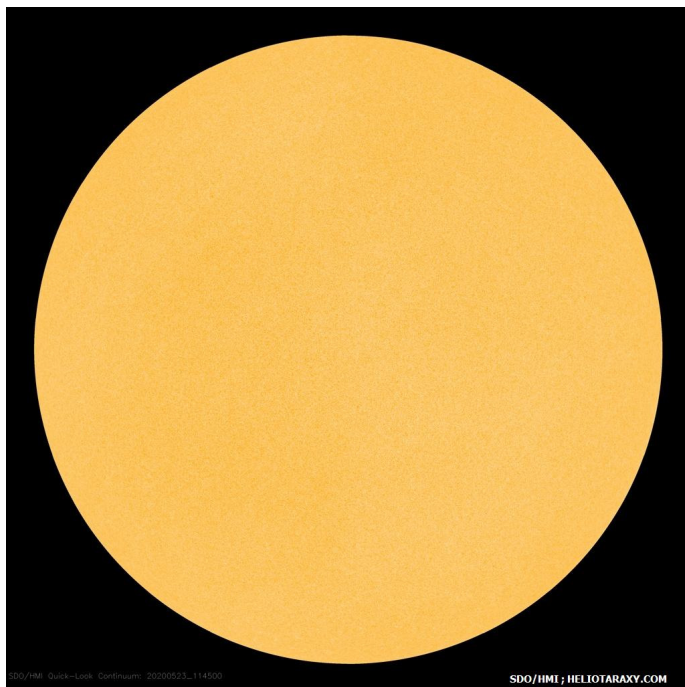
Слънчевият диск на 23 май 2020г (SDO/HMI)
