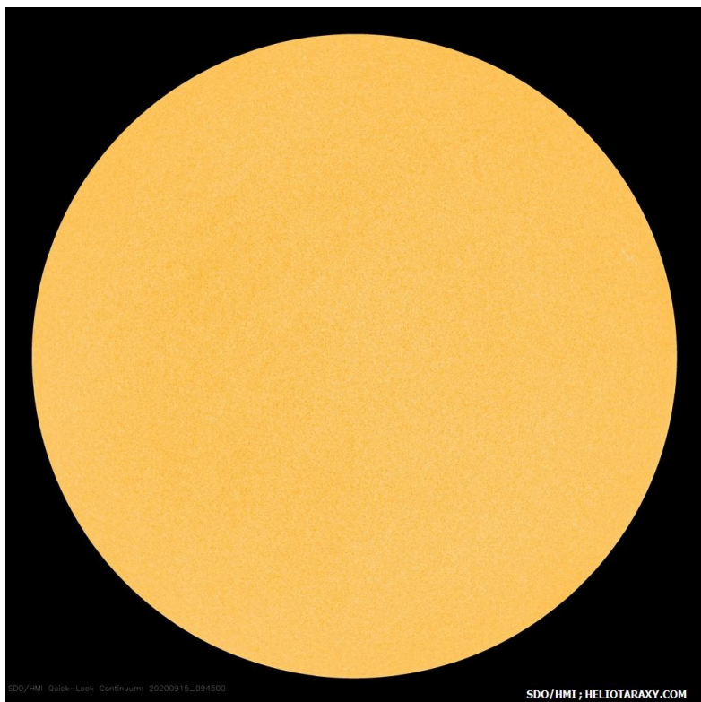
Слънчевият диск на 15 септември 2020г (SDO/HMI)
